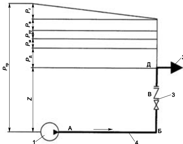
1 — водопитатель; 2 — ороситель; 3 — узел управления; 4 — подводящий трубопровод
